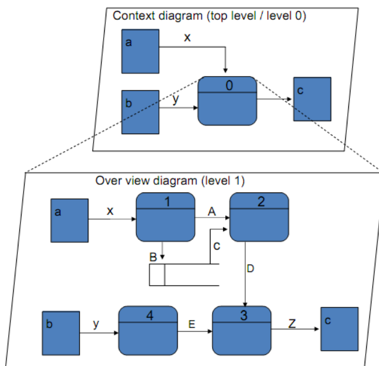
Gambar 11. Pembuatan DFD
